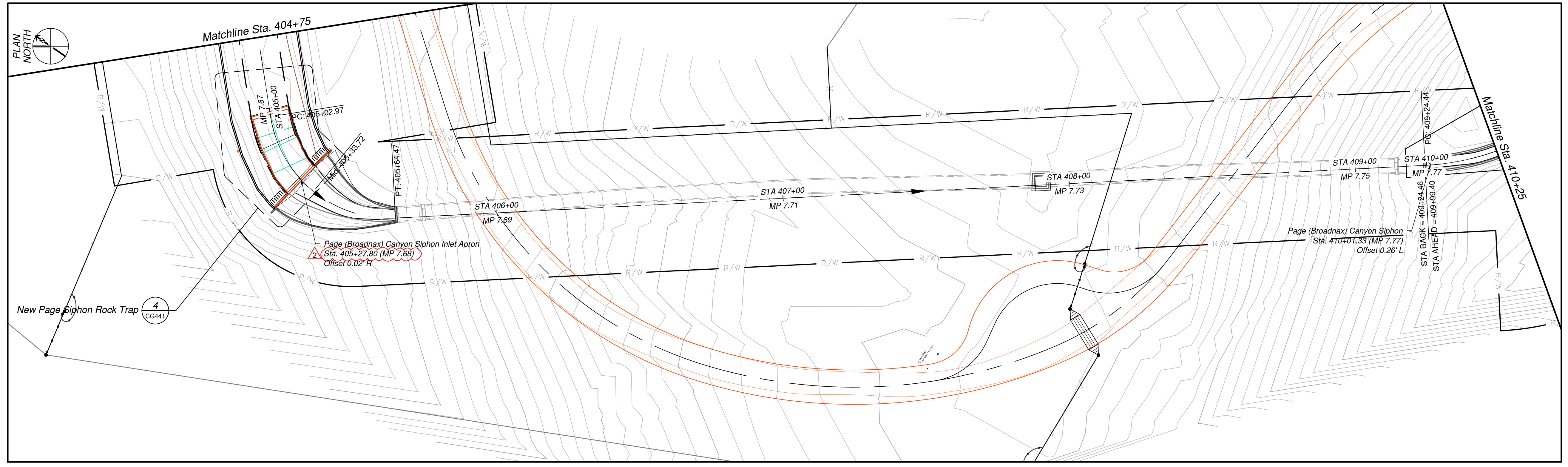
PARTIAL PLAN STA. 404+75 (MP 7.67) TO STA. 410+25 (MP 7.77) 0 10' 20' 40' HORIZONTAL GRID SCALE: 1"=20'
